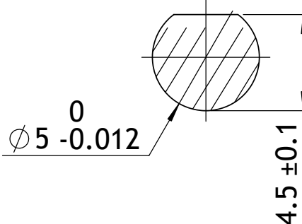
视图 K-K
