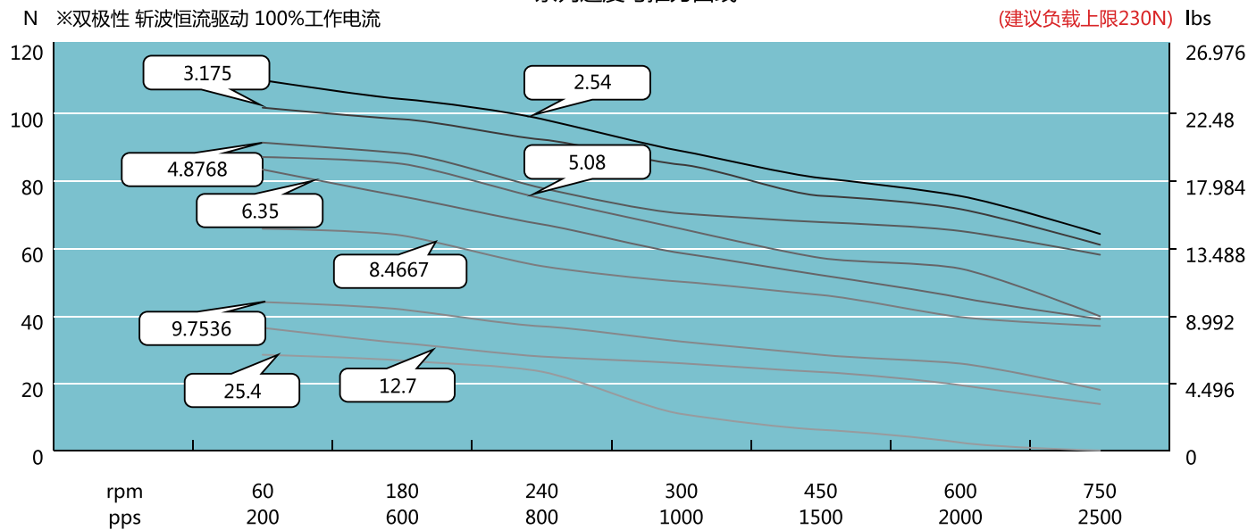
35-234系列速度与推力曲线
