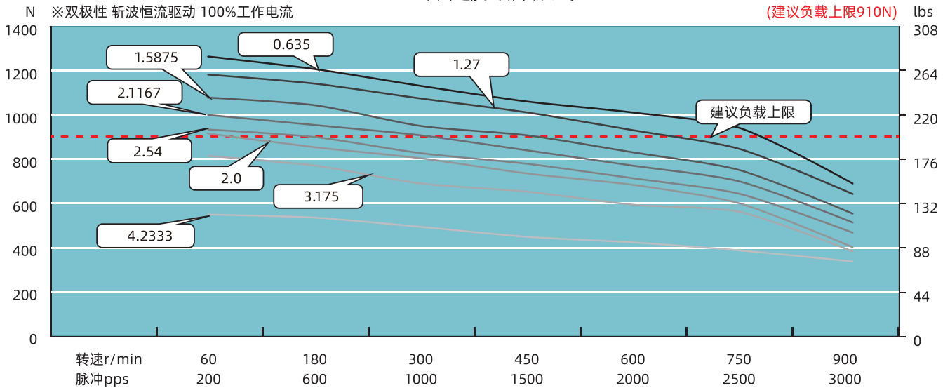
57-265 系列速度与推力曲线
