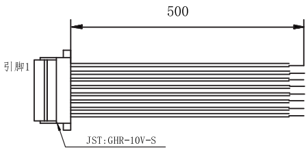
编码器线束图
