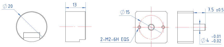
编码器外形图
