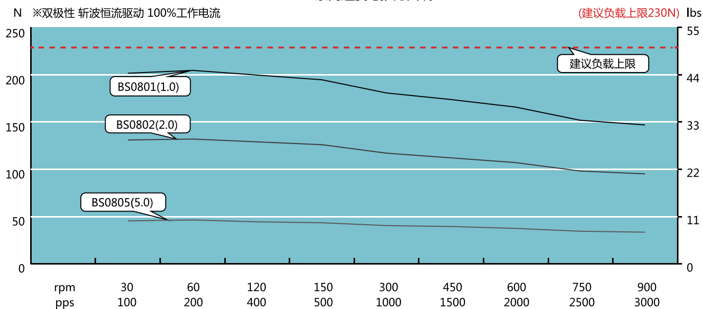
35E234系列速度与推力曲线
