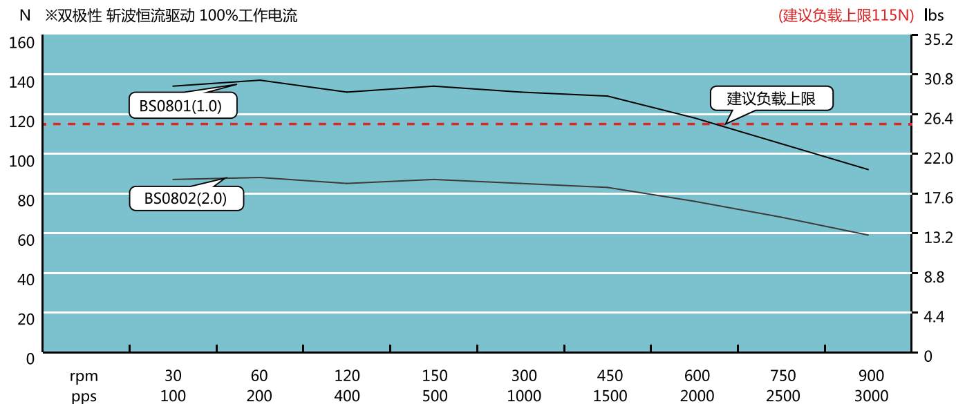
28E234系列速度与推力曲线
