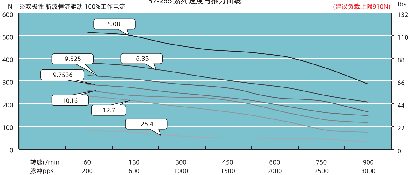
57-265 系列速度与推力曲线
