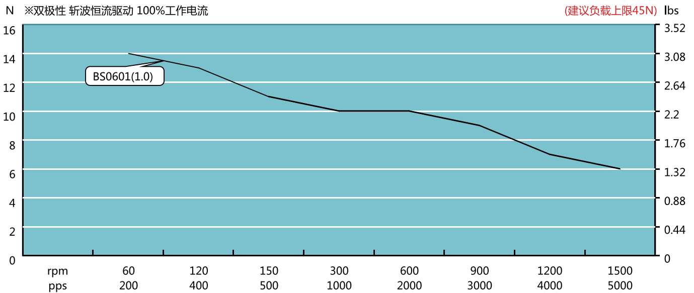
20E228系列速度与推力曲线
