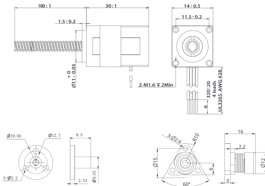
标准螺母
