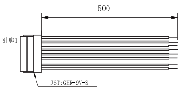
编码器线束图
