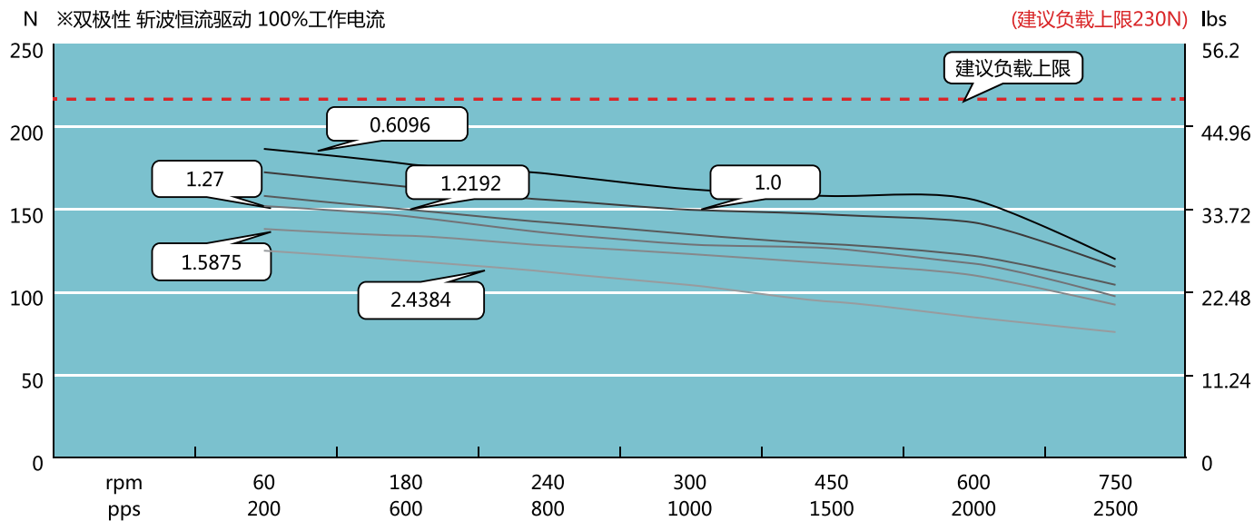
35-234系列速度与推力曲线
