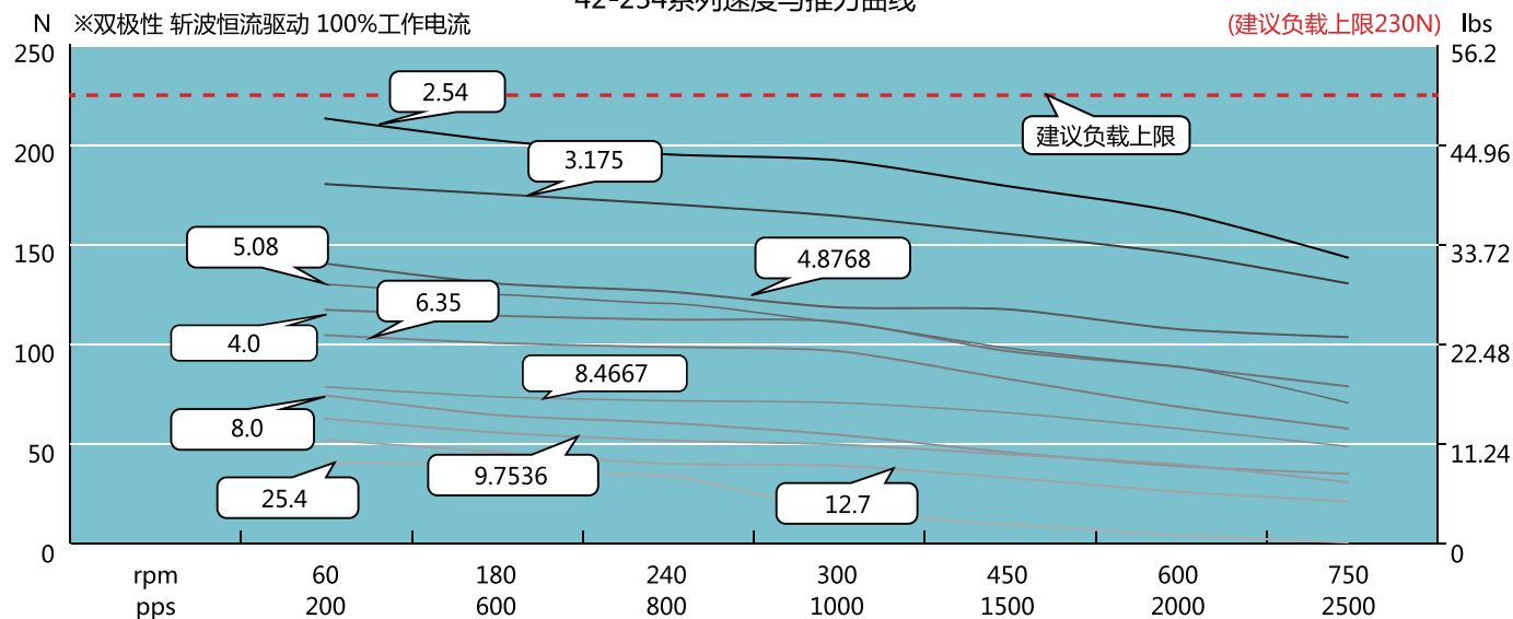
42-234系列速度与推力曲线
