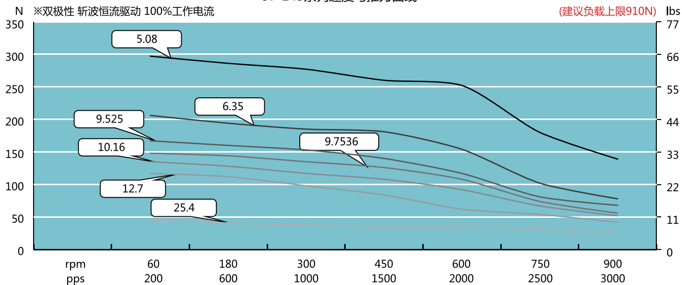
57-245系列速度与推力曲线
