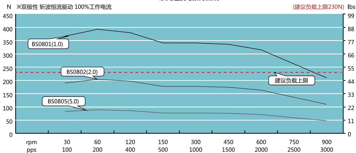
35E247系列速度与推力曲线
