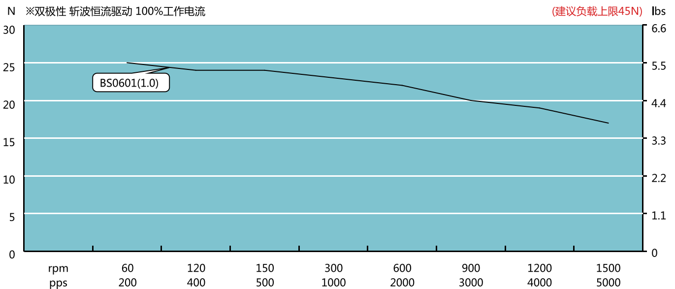
20E238系列速度与推力曲线
