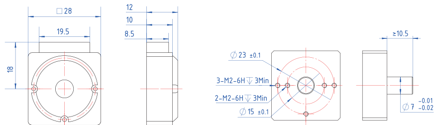
编码器外形图
