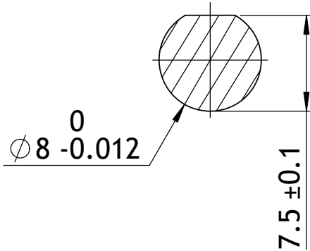
视图 P-P
