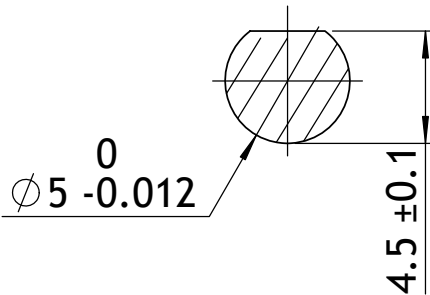
视图P-P
