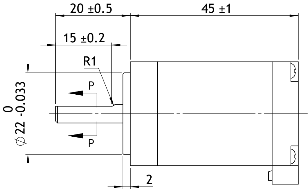
视图P-P
