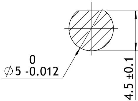
视图P-P
